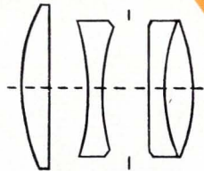
COLOR-SKOPAR 1:3,5
